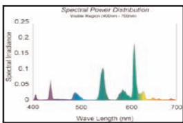
OPTIONAL TL83 (3000K) Green bias,
