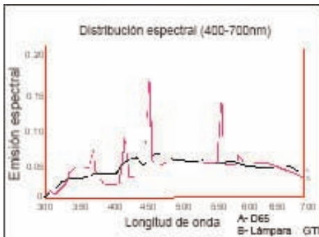
Lámpara ColorMatcher de D65
