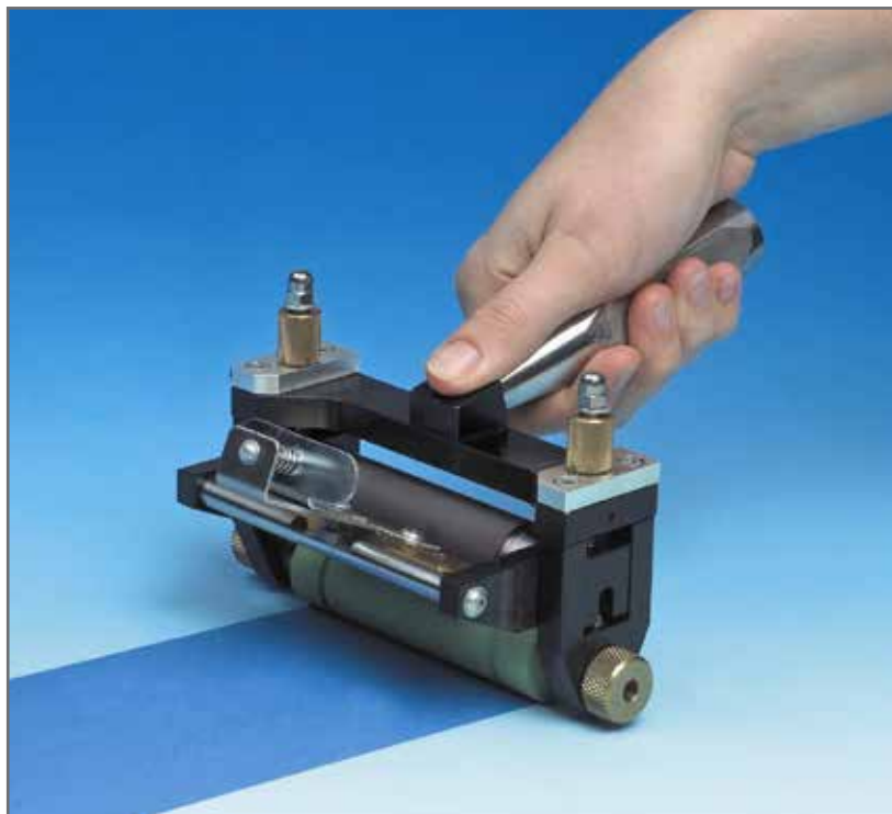
Esiproof con control de la presión por resorte cargado
