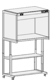
C28-A Model: CMB-2028/FS C40-A Model: CMB-2540/FS C52-A Model: CMB-3052/FS C64-A Model: CMB-3064/FS
